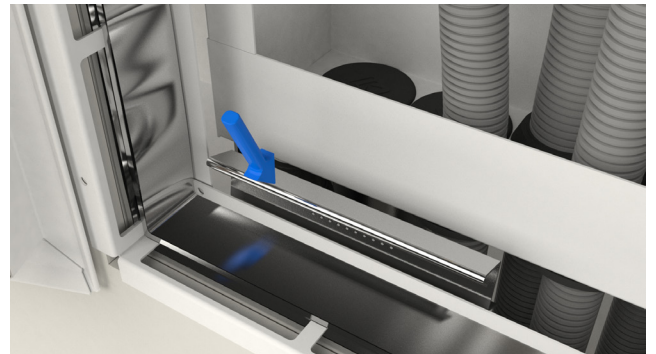
Aseta kiinnityslevyt kehyksen päälle ja paina ne kipsilevyn takaosaan.
