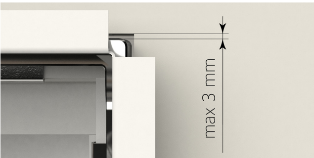
Asennusreiän reunan ja kehyksen väli saa olla enintään 3 mm.
